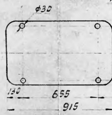
Расположение фунда станка с мет
