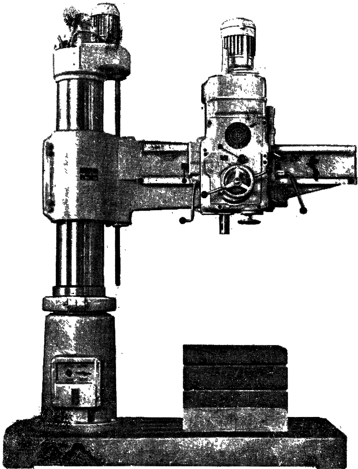
Рис. 1. Радиально-сверлильный станок модели 2А53.
