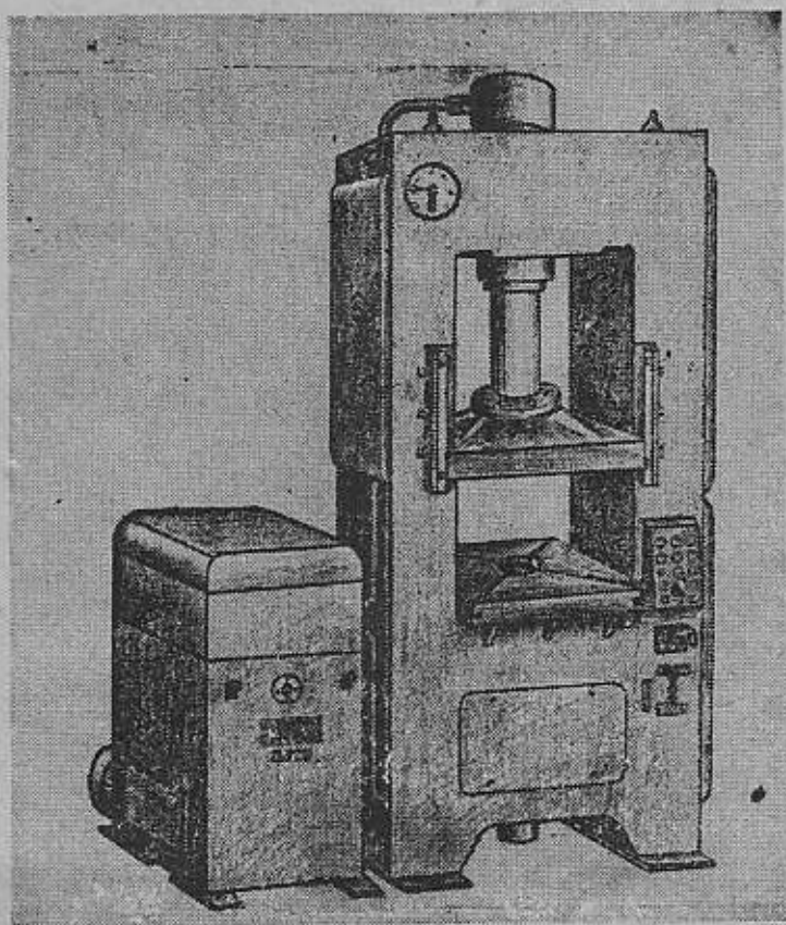
ПРЕСС ГИДРАВЛИЧЕСКИЙ ДЛЯ ПЛАСТМАСС модели Д2428
