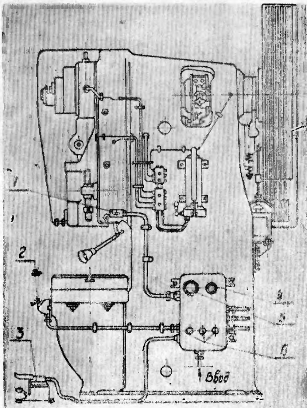
Рис. 1. Общий вид пресса. 1 и 2 — кнопки включения электродвигателя; 3 — педаль ножного включения; 4 — выключатель местного освещения; 5 — вводный выключатель; 6 — сигнальные лампы.
