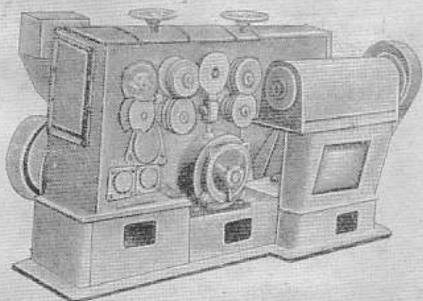
Рис. 1. Общий вид станка СМЖ-142А
