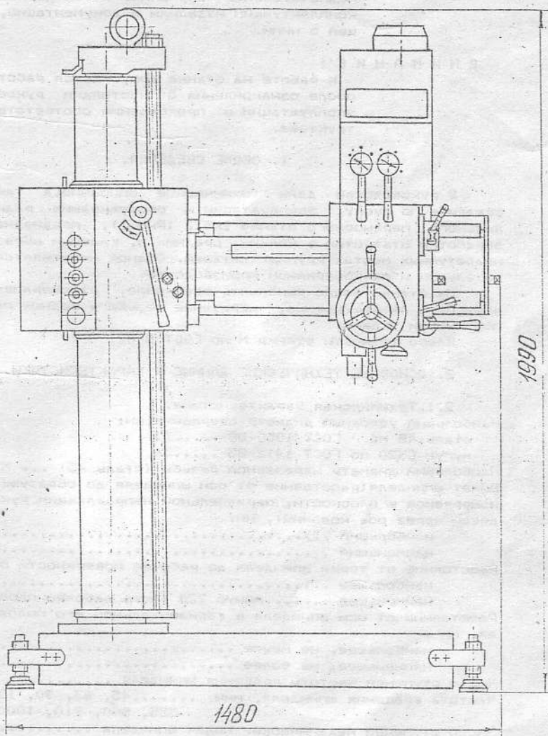
Рис.1. Станок радиально-сверлильный
