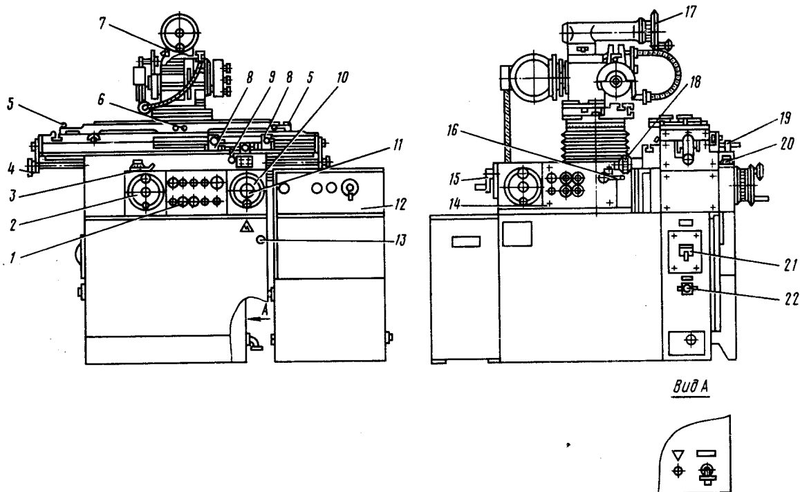
Рис. 2. Расположение органов управления
