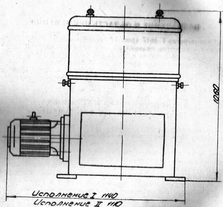
Рис. 1. Общий вид гидроагрегата
