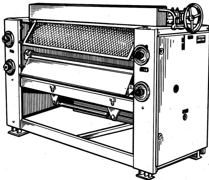
Рис. 1. Станок клеенаносящий вальцовый модели КВ
