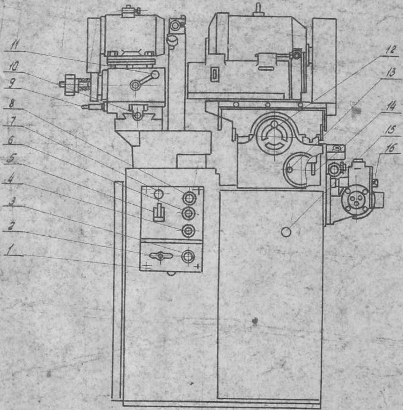
Рис. 4. Органы управления станком
