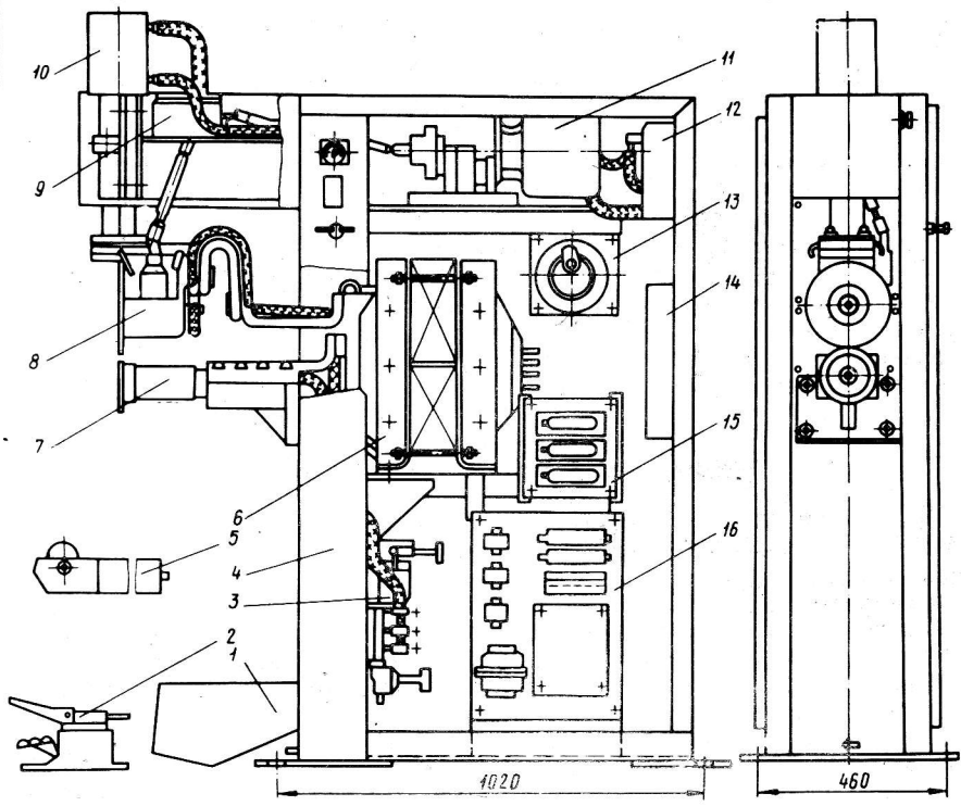
Рис. 1. Общий вид машины
