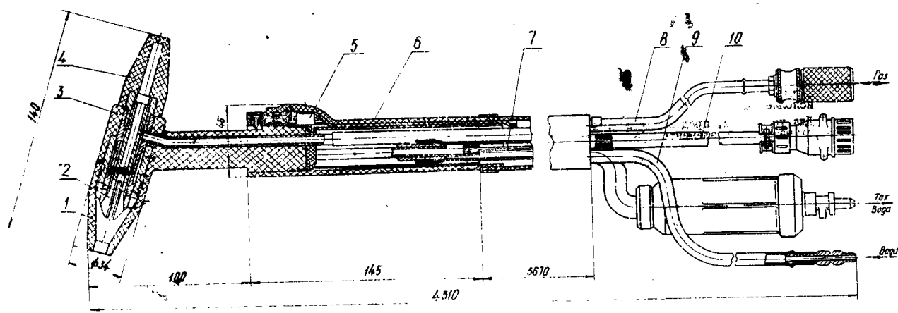
Рис. 4. Горелка средняя ГР-6
