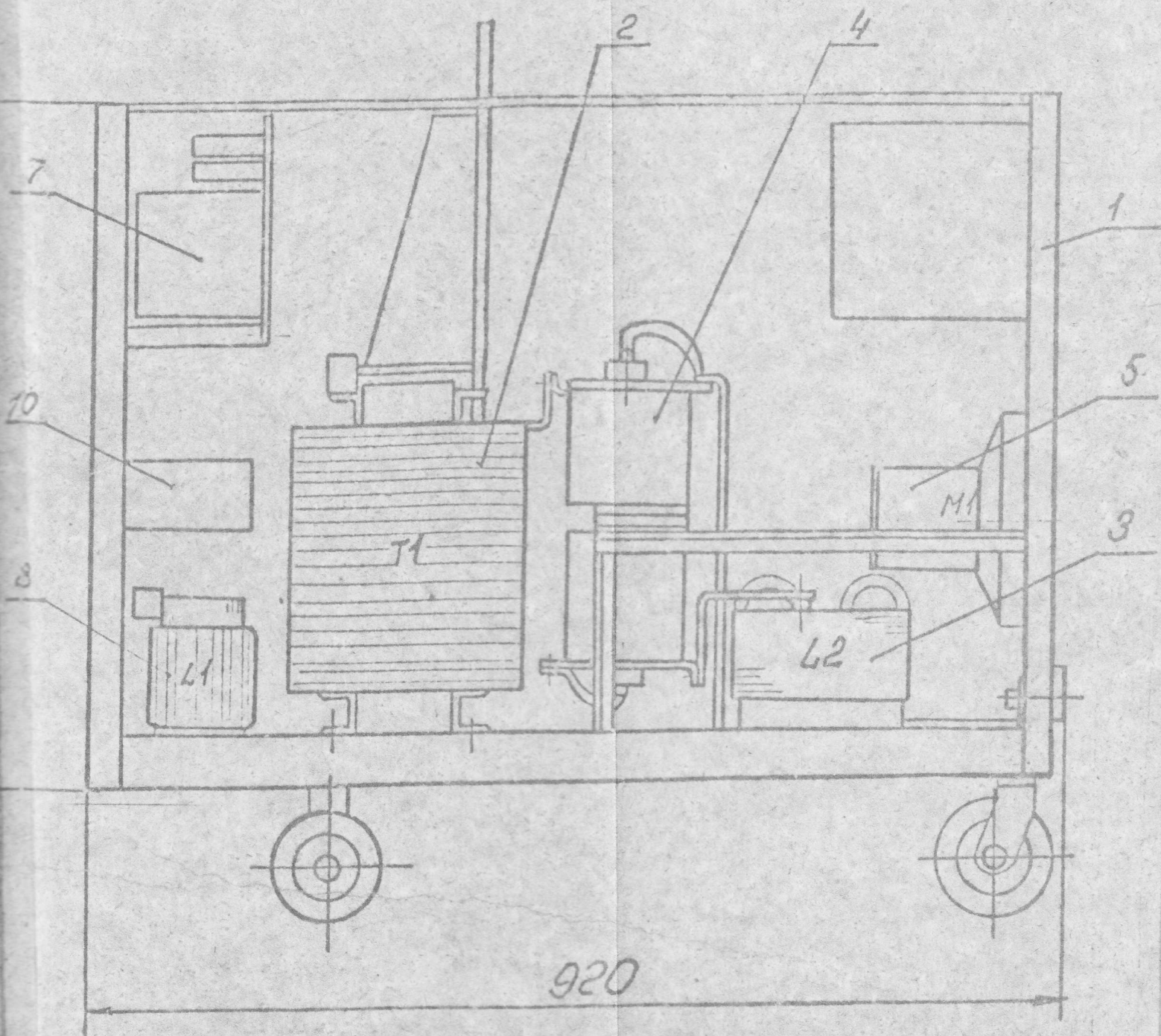
Рис. 1. Выпрямитель универсальный для сварки неплавящимся электродом модели ВСВУ-400.
